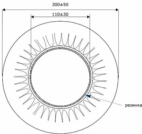
Рис.1. Основные размеры изделия мед. шапочка «Шарлотта»
